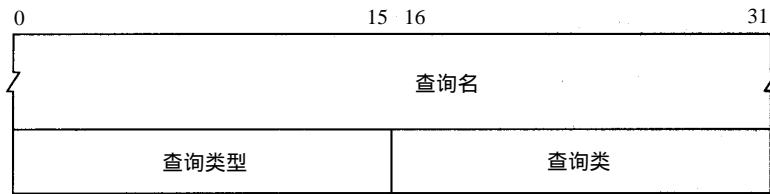
图14-5 DNS查询报文中问题部分的格式
