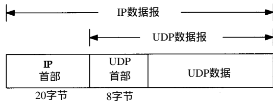
图11-1 UDP封装
