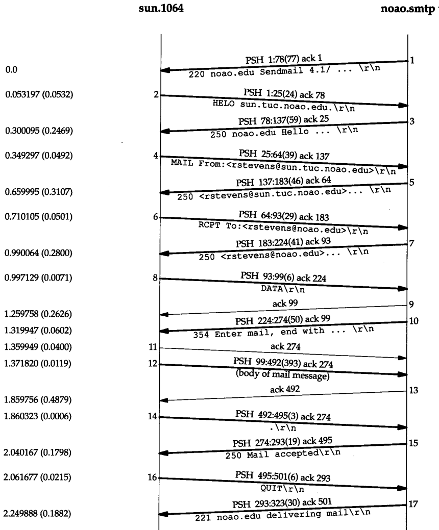
图28-2 基本SMTP邮件交付
