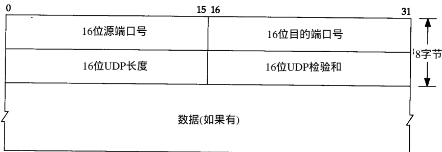
图11-2 UDP首部
