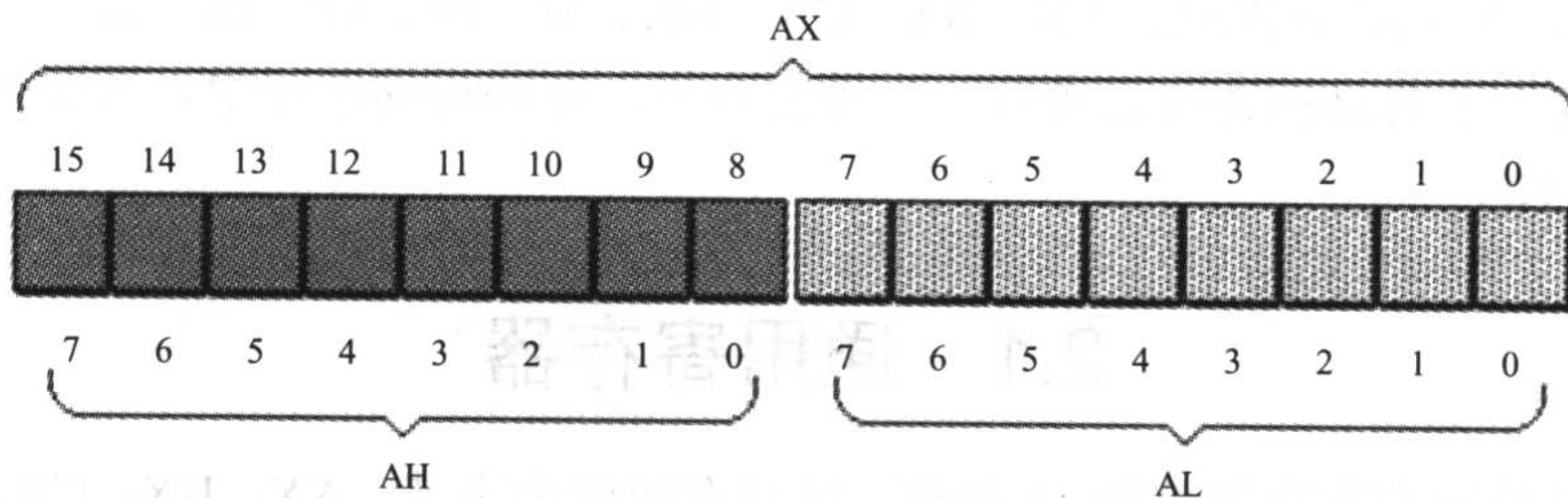
图 2.3 16 位寄存器分为两个 8 位寄存器
