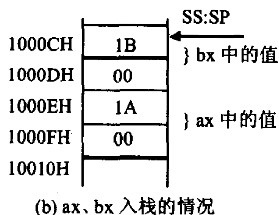
图 3.15 栈的情况示意(1)
