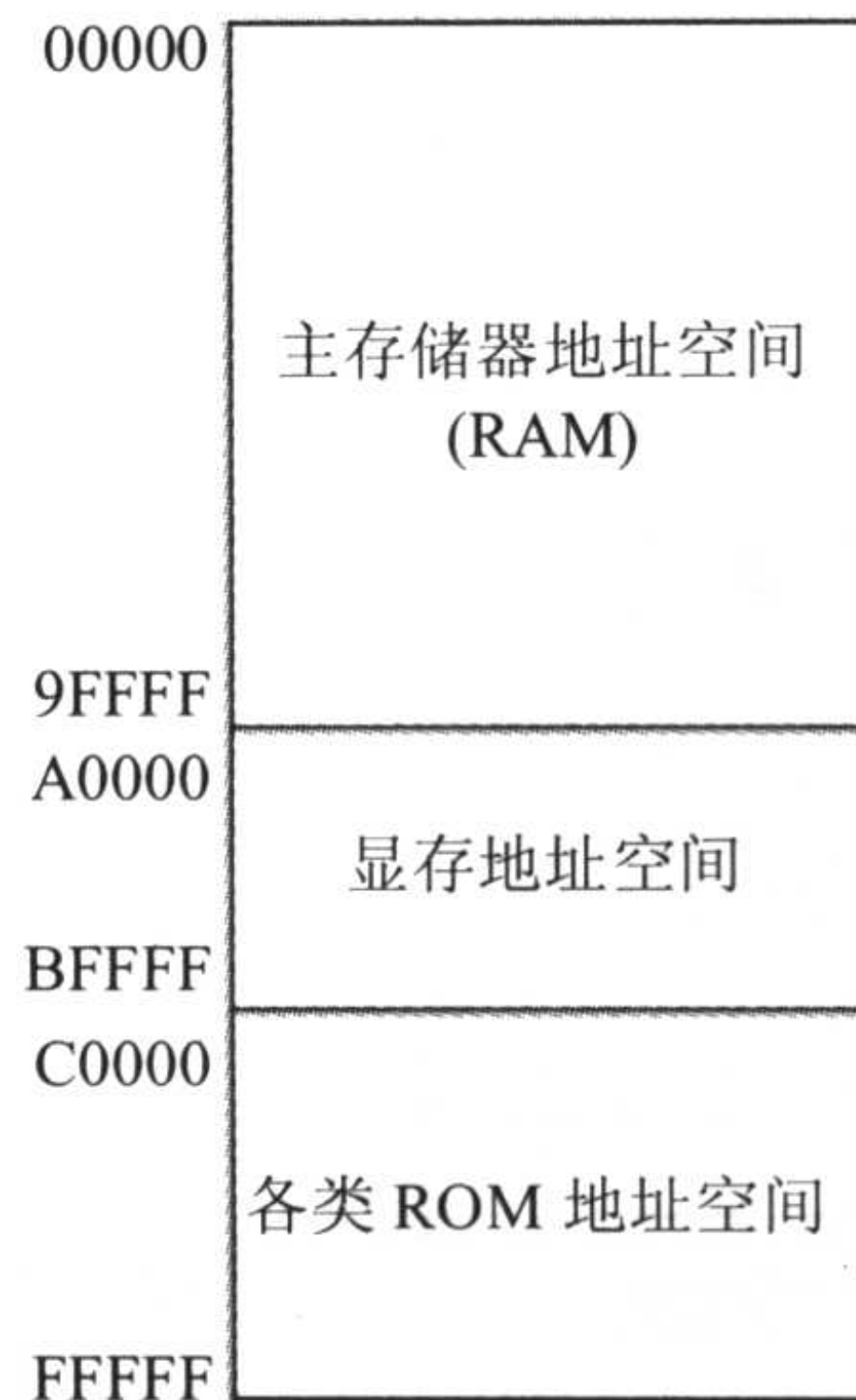
图 1.9 8086PC 机内存地址空间分配
