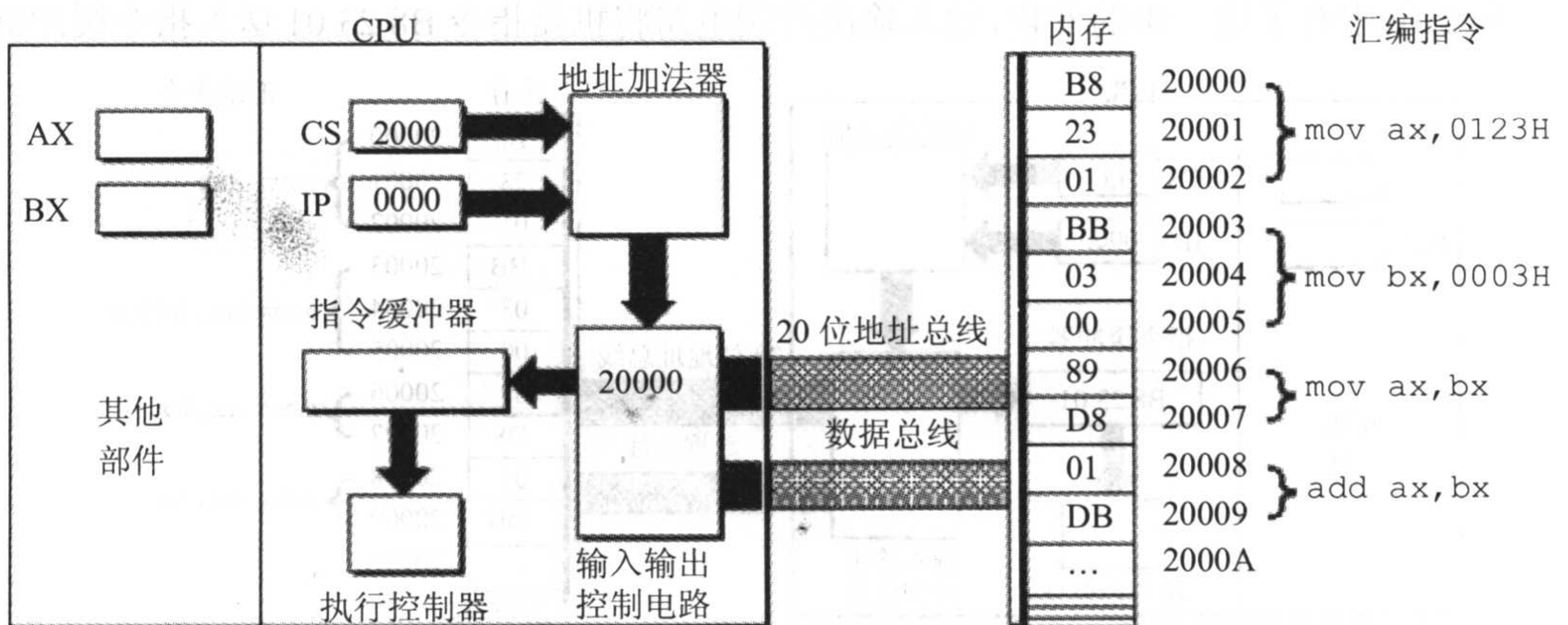
图 2.13 物理地址被送入输入输出控制电路
