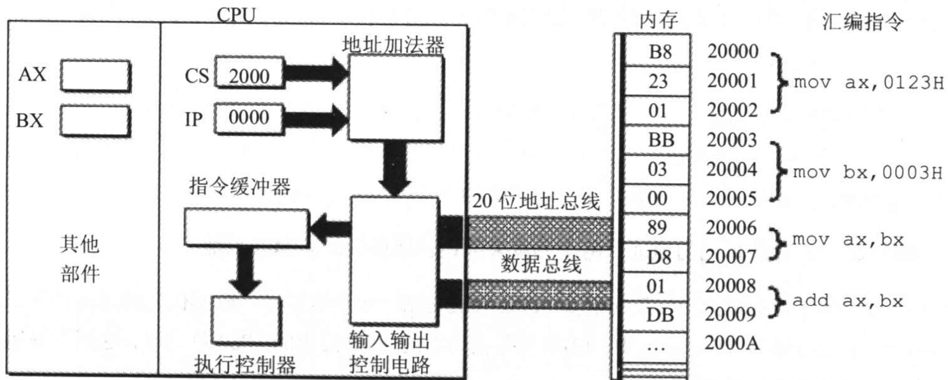
图 2.10 8086PC 读取和执行指令的相关部件
