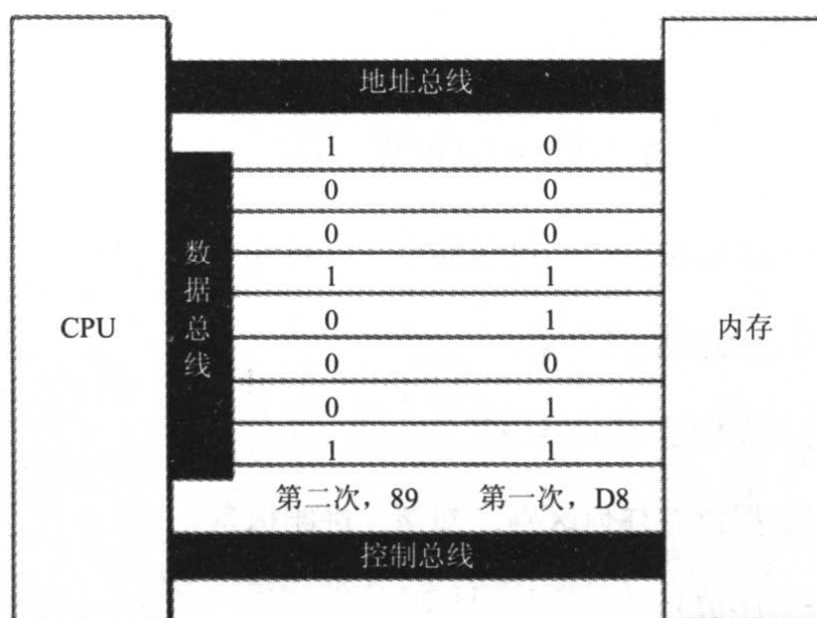
图 1.5 8 位数据总线上传送的信息
