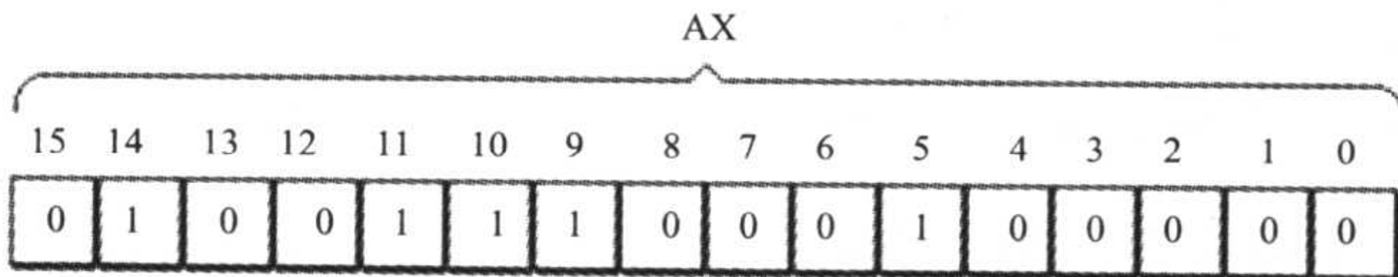
图 2.2 16 位数据在寄存器中的存放情况
