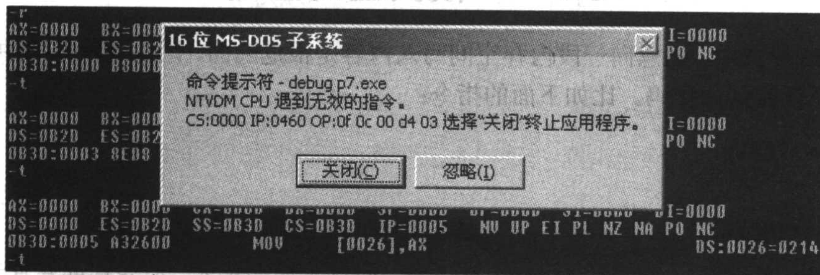
图 5.19 改写 0:0026 处存放的重要系统数据
