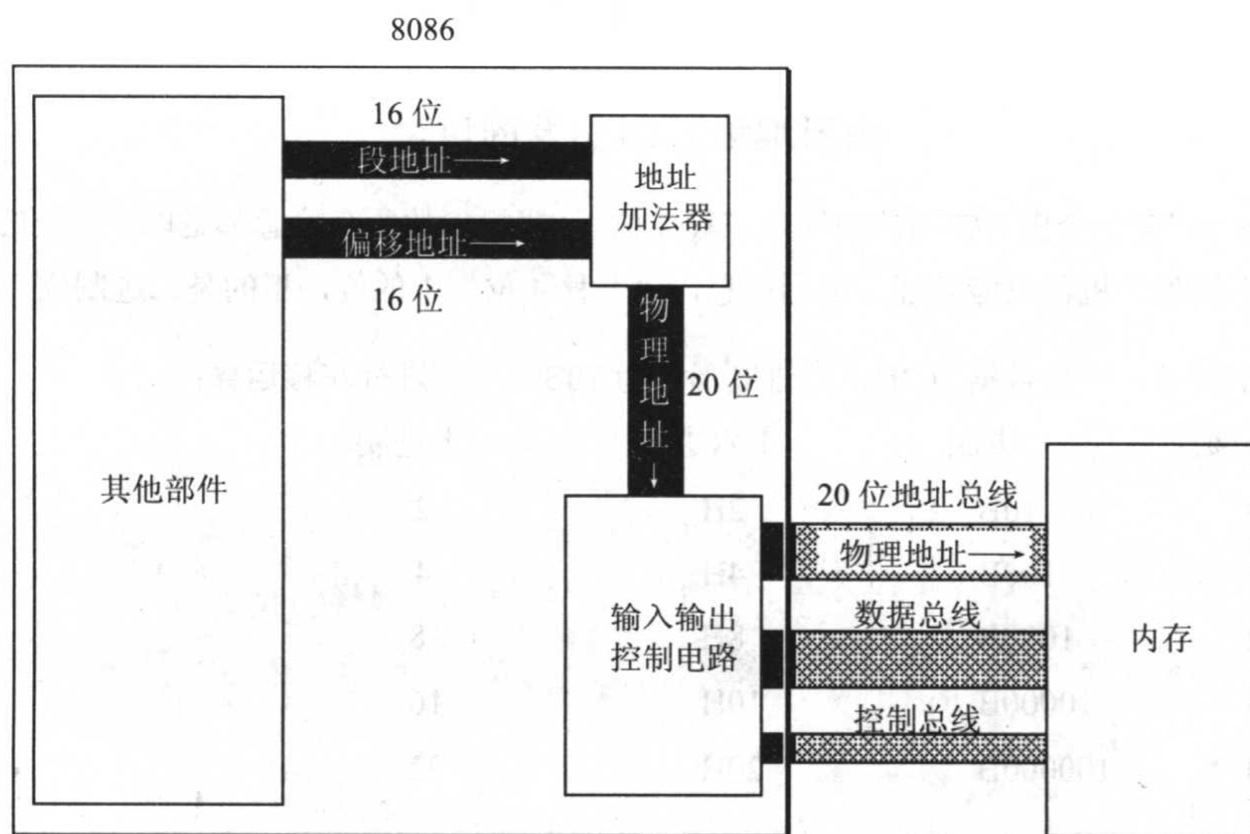
图 2.6 8086CPU 相关部件的逻辑结构
