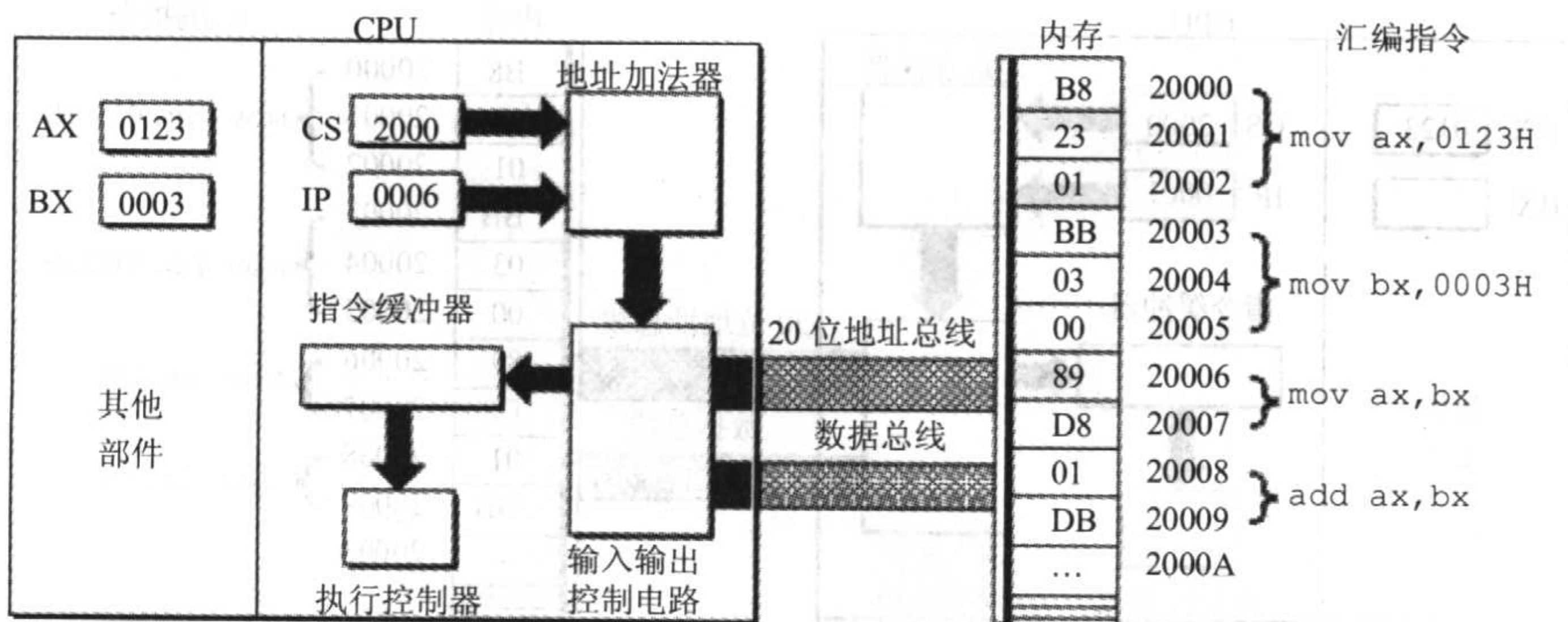
图 2.22 第二条指令执行情况
