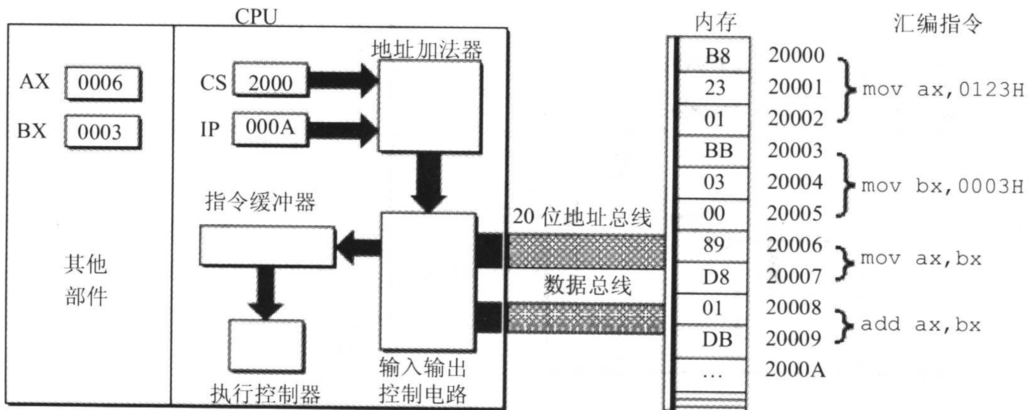
图 2.26 第四条指令执行情况
