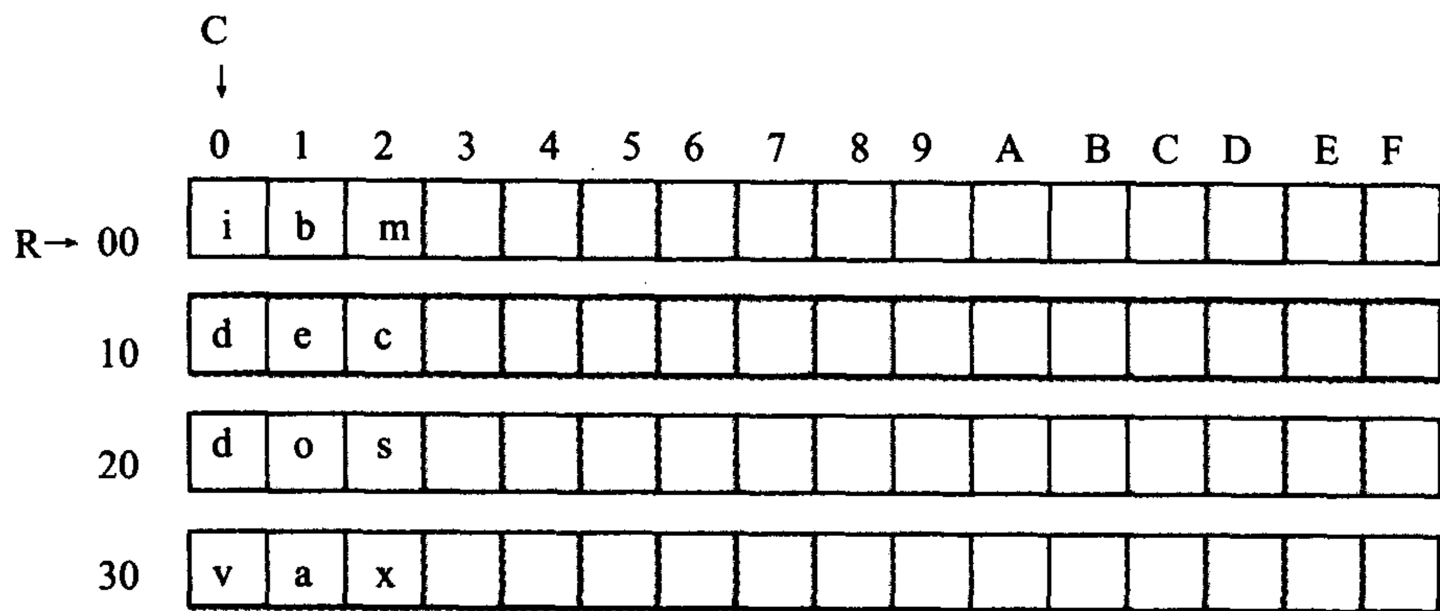
图 7.3 datasg 中数据的存储结构
