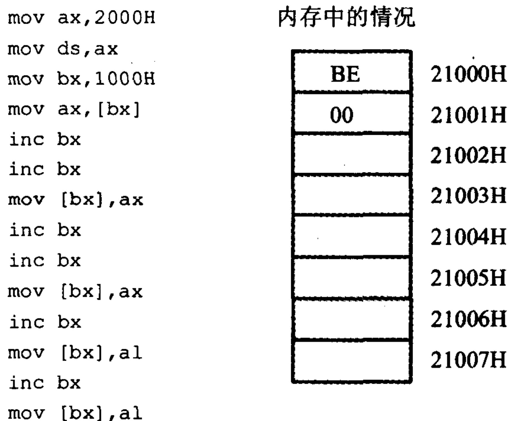
图 5.1 问题 5.1 程序和内存示意
