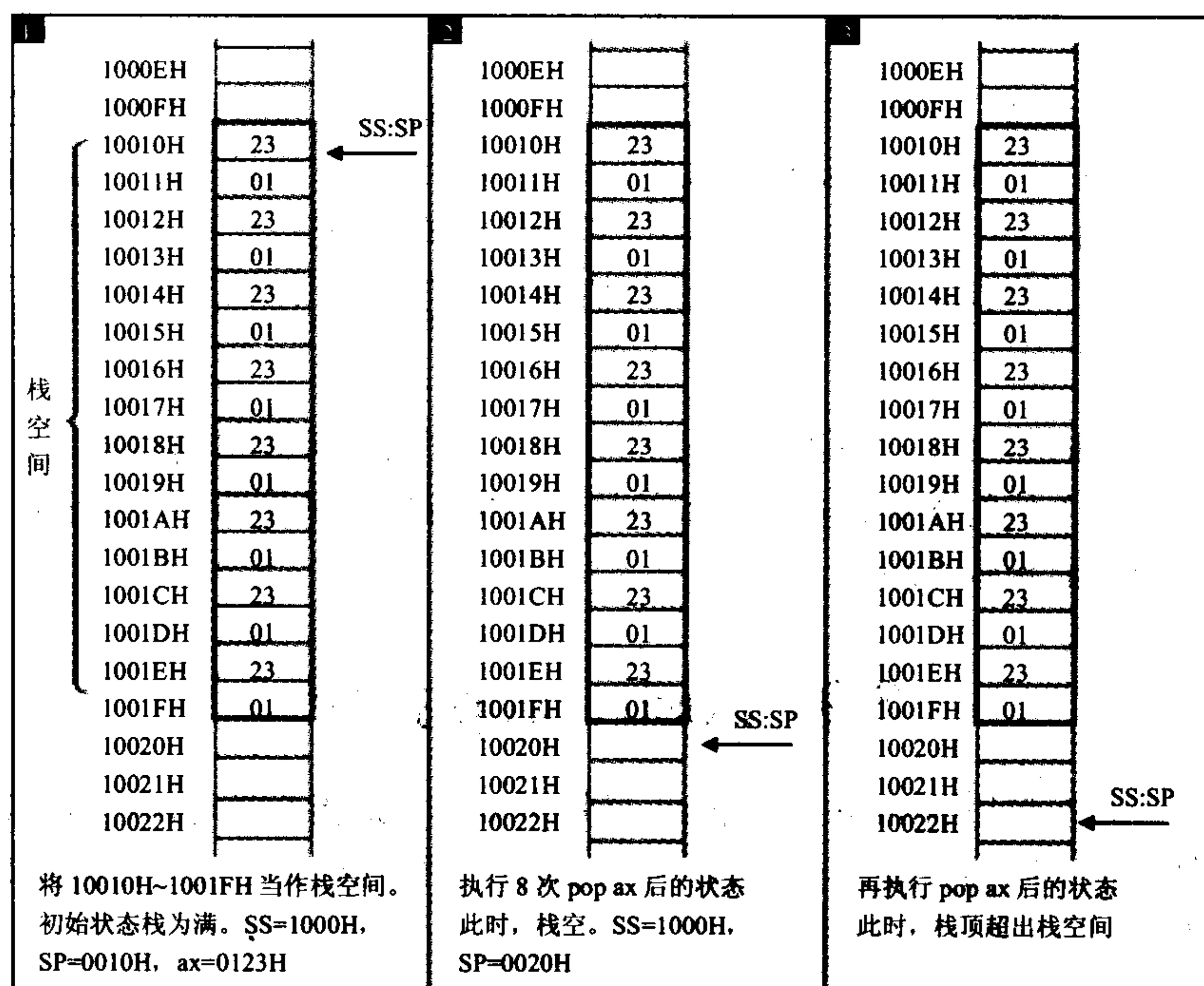
图 3.14 执行 pop 指令后栈顶超出栈空间
