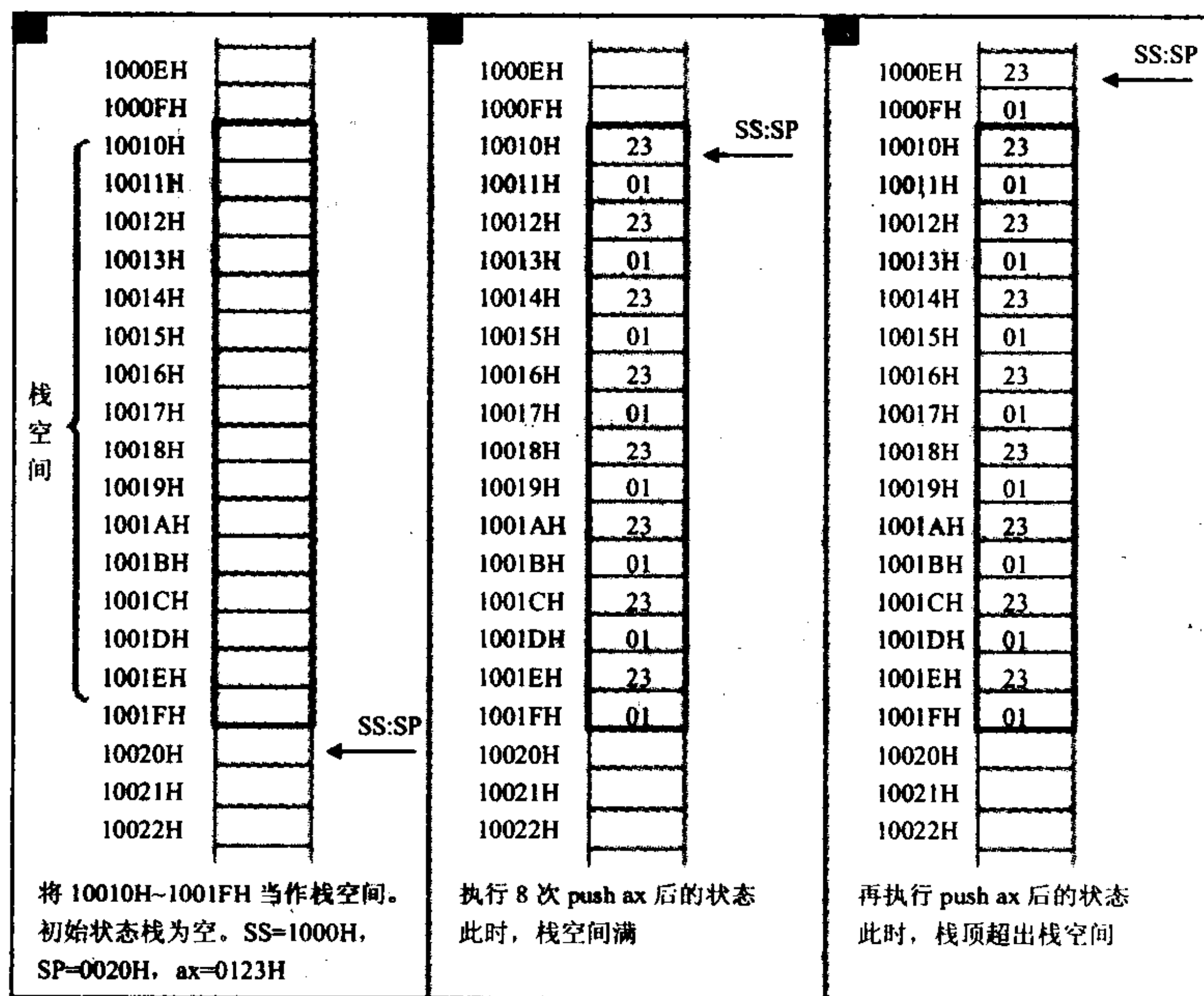
图 3.13 执行 push 后栈顶超出栈空间
