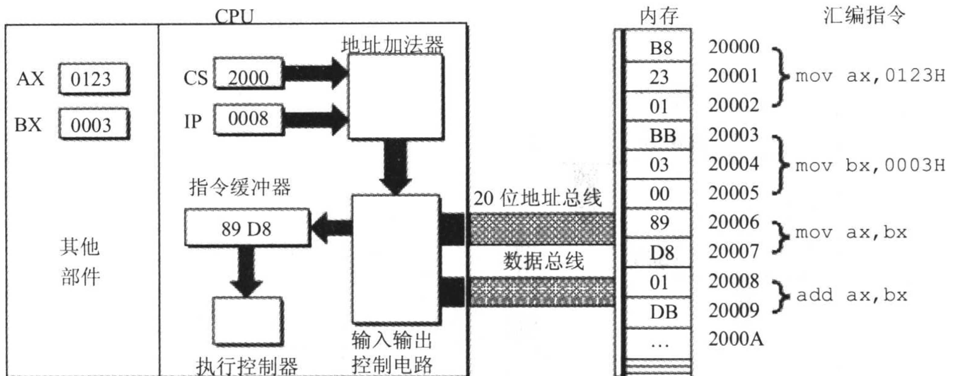
图 2.23 第三条指令被读入指令缓冲器
