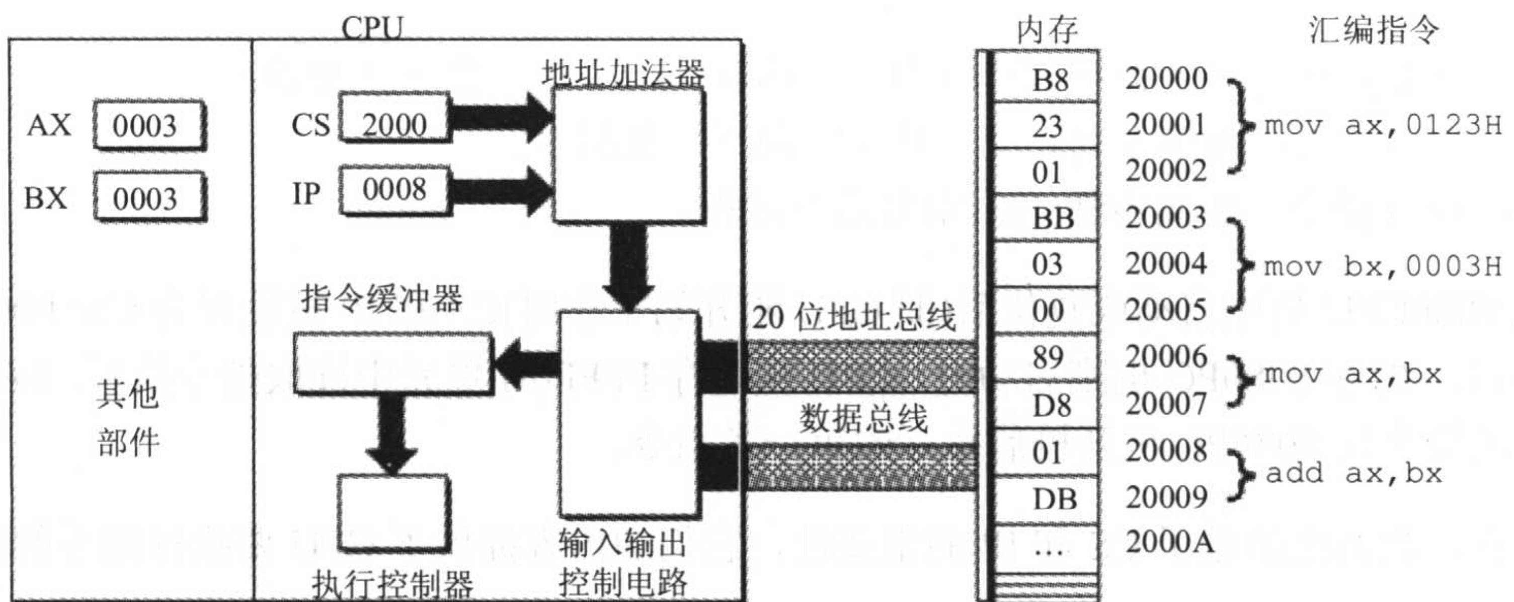
图 2.24 第三条指令执行情况
