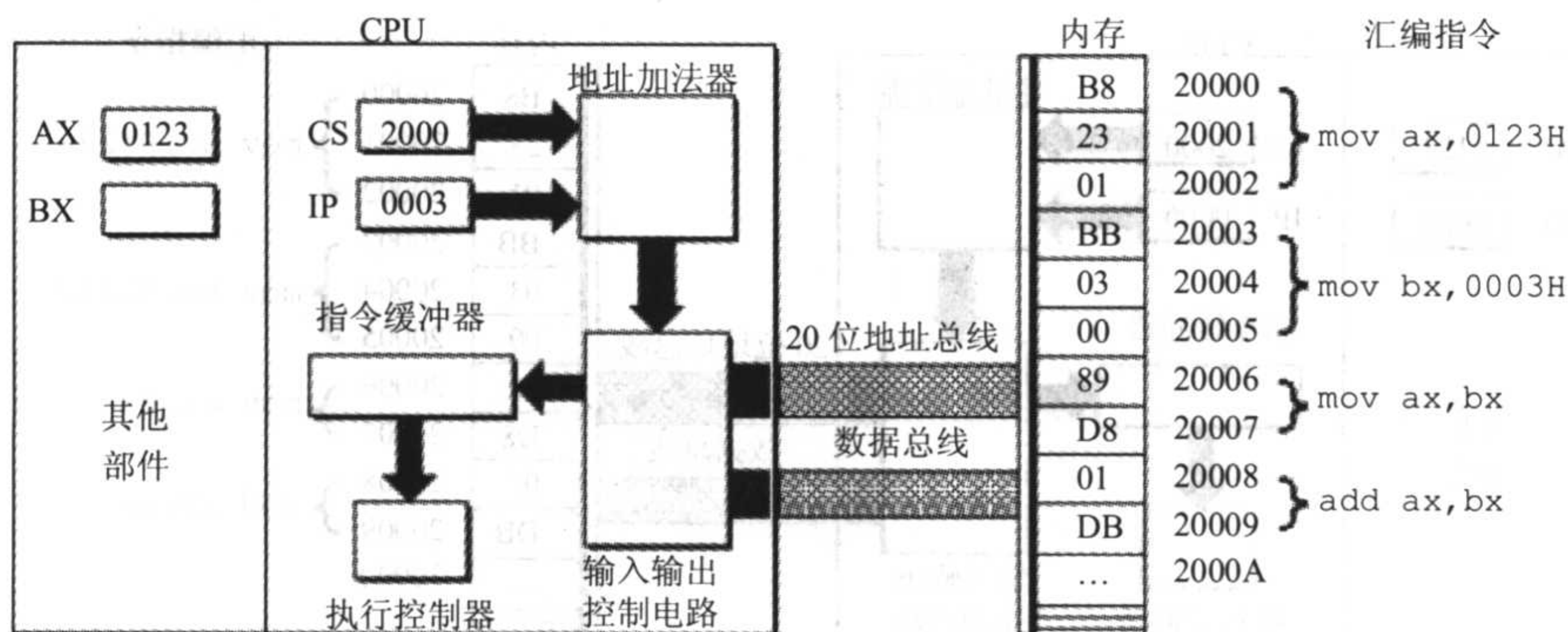
图 2.19 指令执行结果
