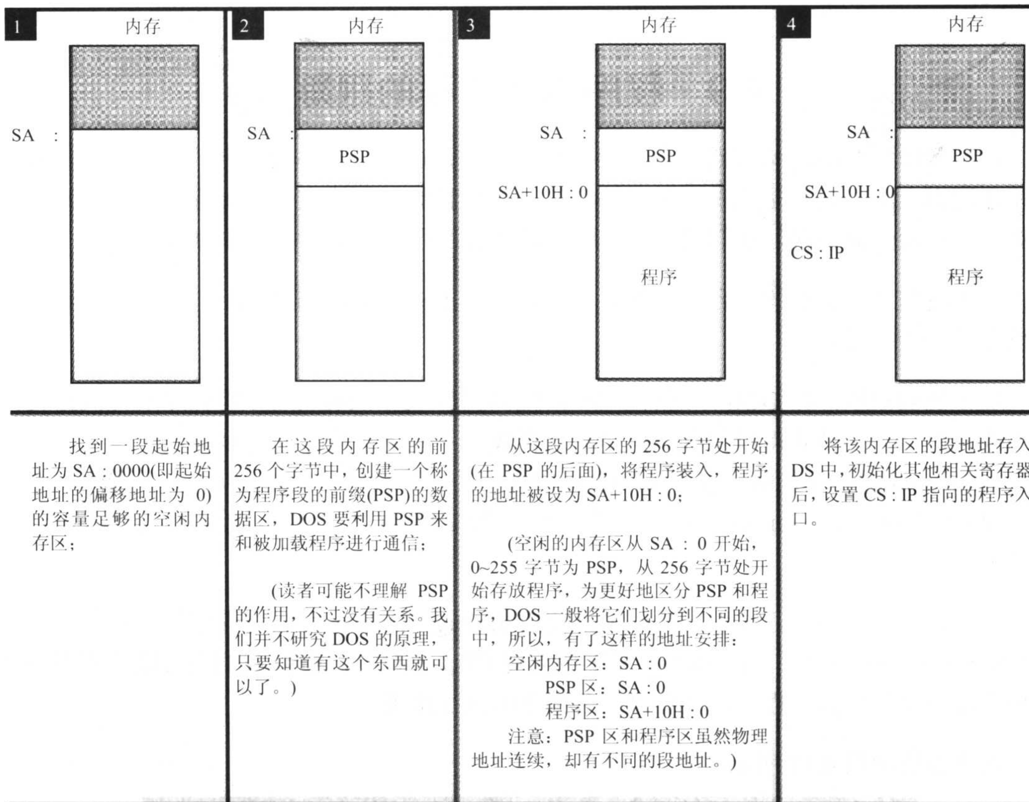
图 4.20 EXE 文件中程序的加载过程
