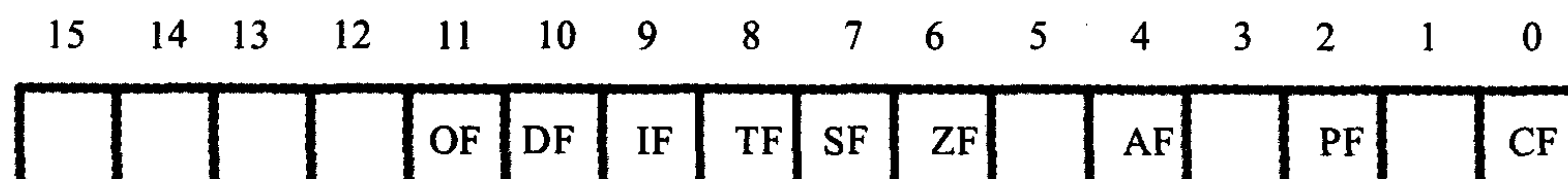
图 11.1 flag 寄存器各位示意
