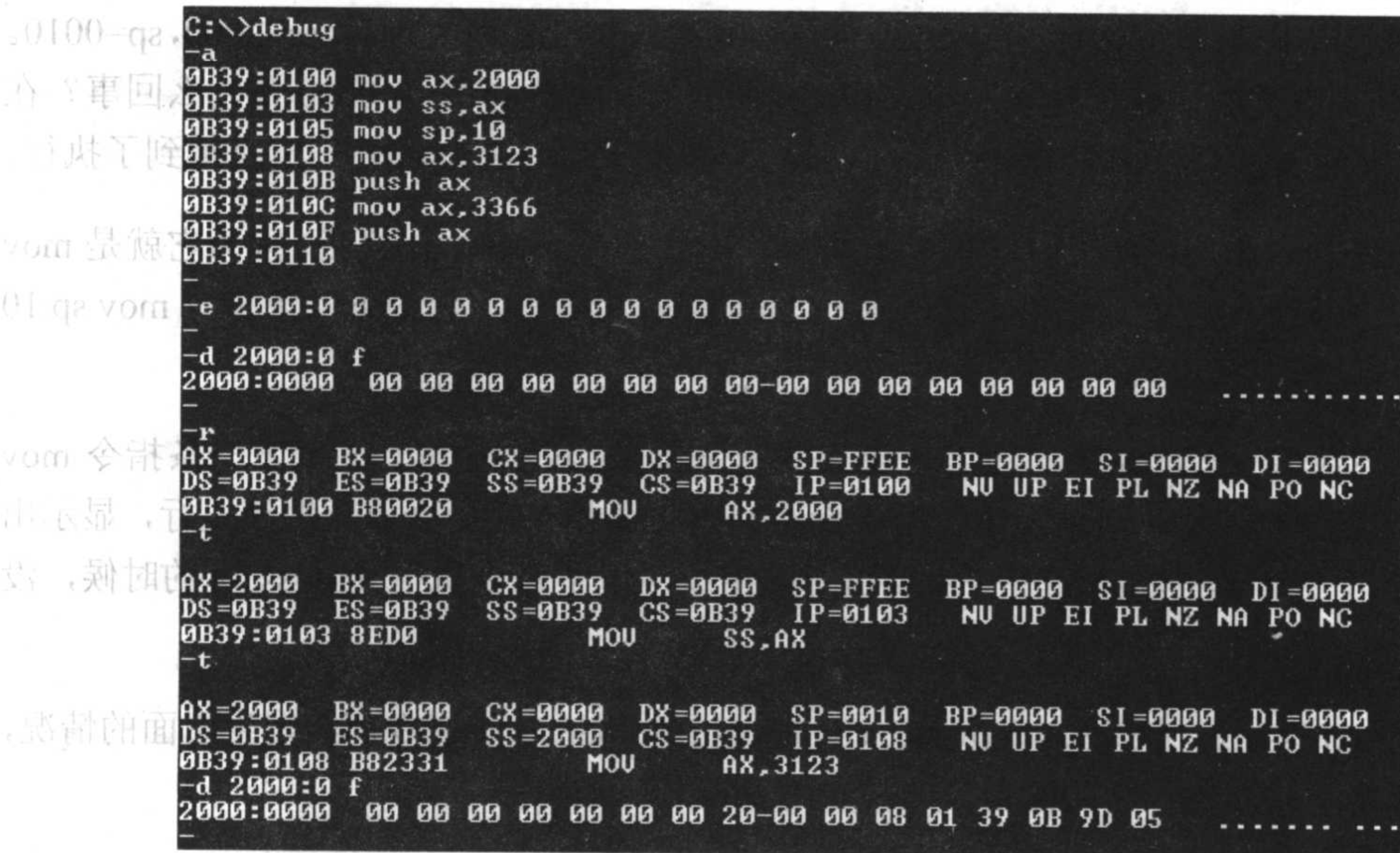
图 3.19 用 Debug 进行实验的示例
