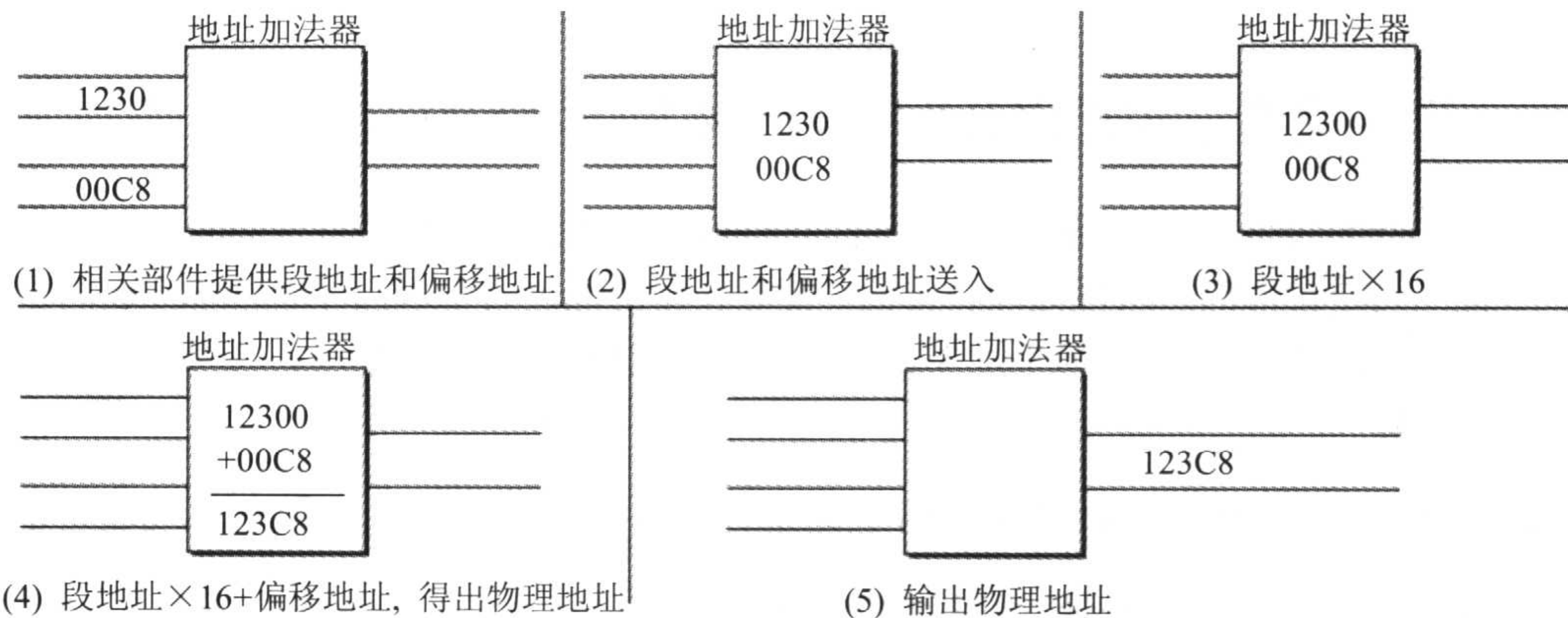
图 2.7 地址加法器的工作过程
