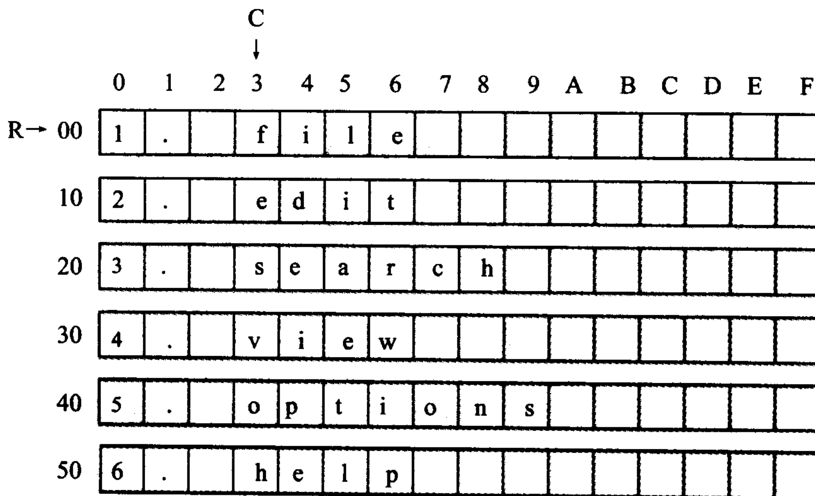
图 7.2 datasg 中数据的存储结构
