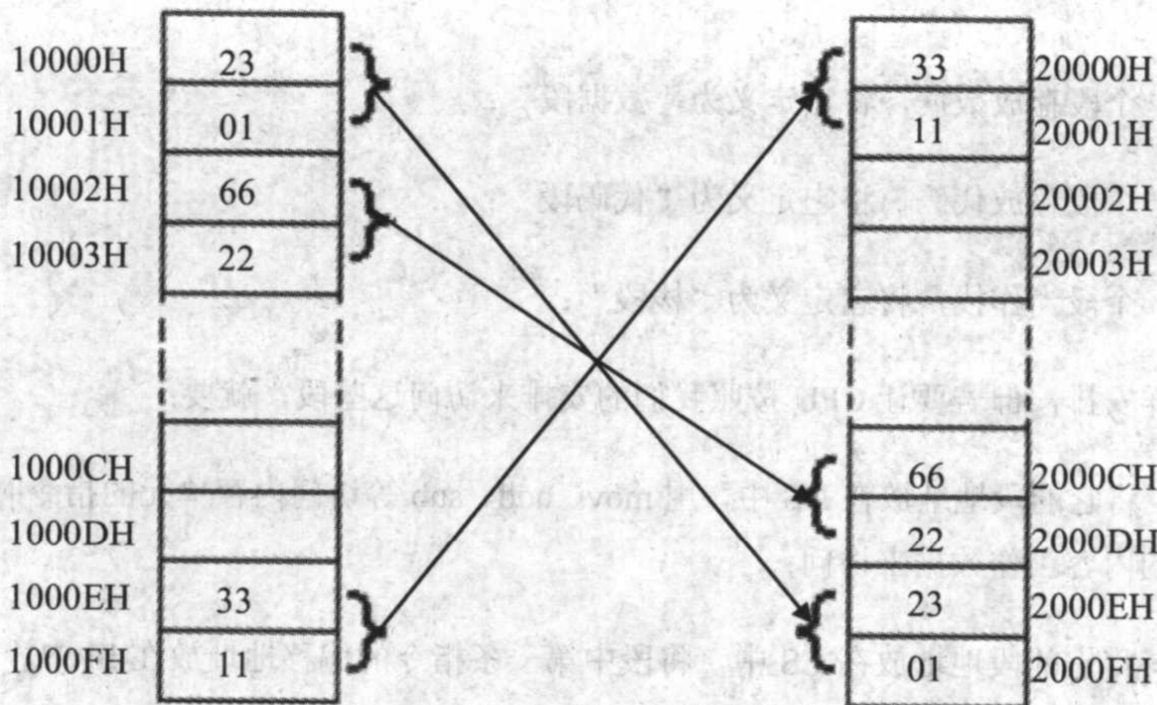
图 3.17 逆序拷贝示意
