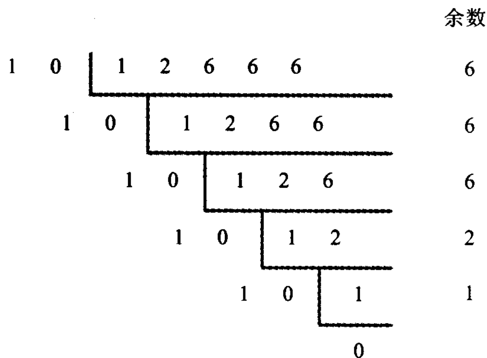
图 10.2 除 10 取余法示意
