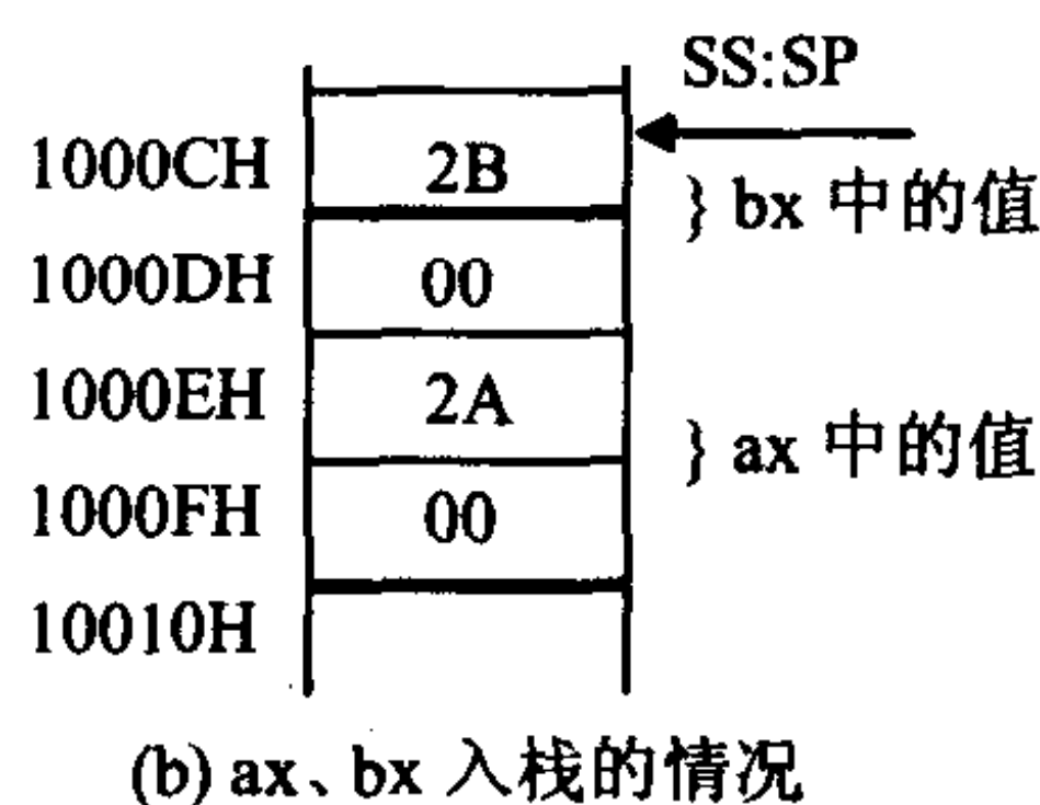
图 3.16 栈的情况示意(2)
