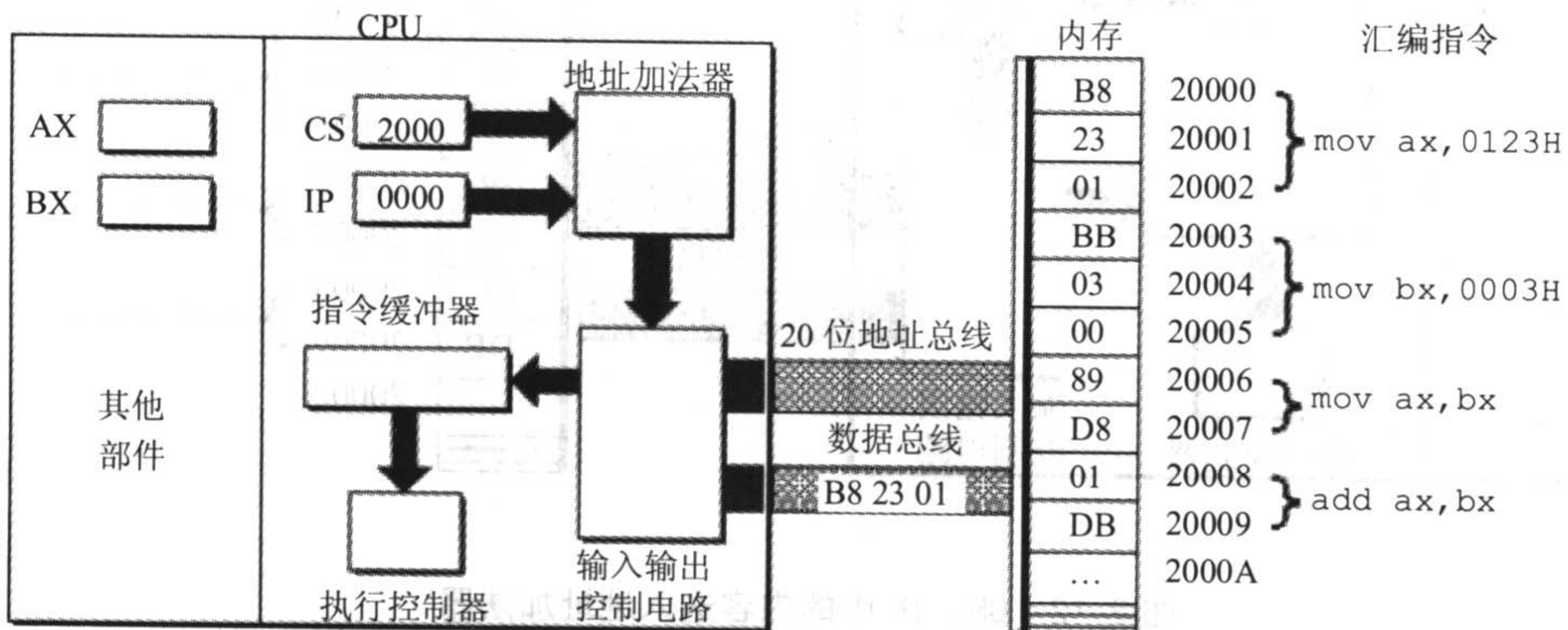
图 2.15 机器指令被送入 CPU
