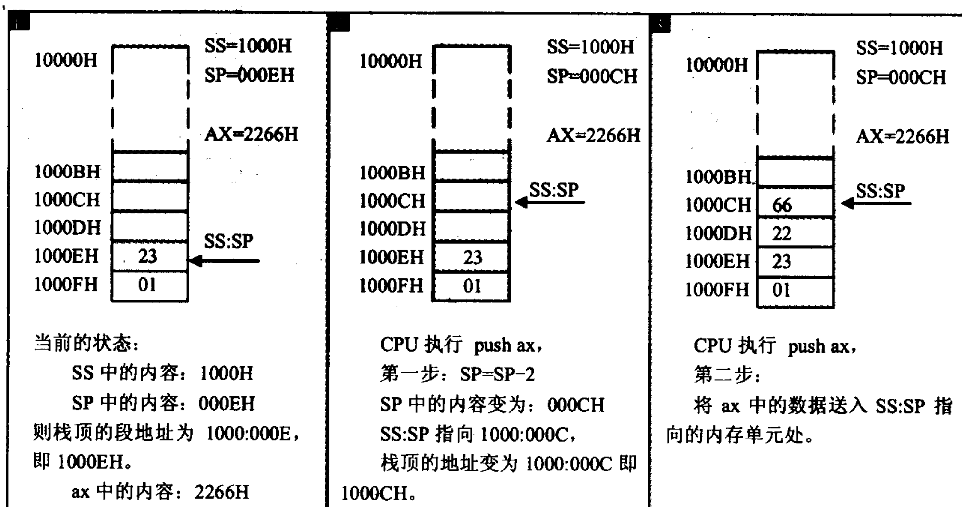
图 3.10 push 指令的执行过程
