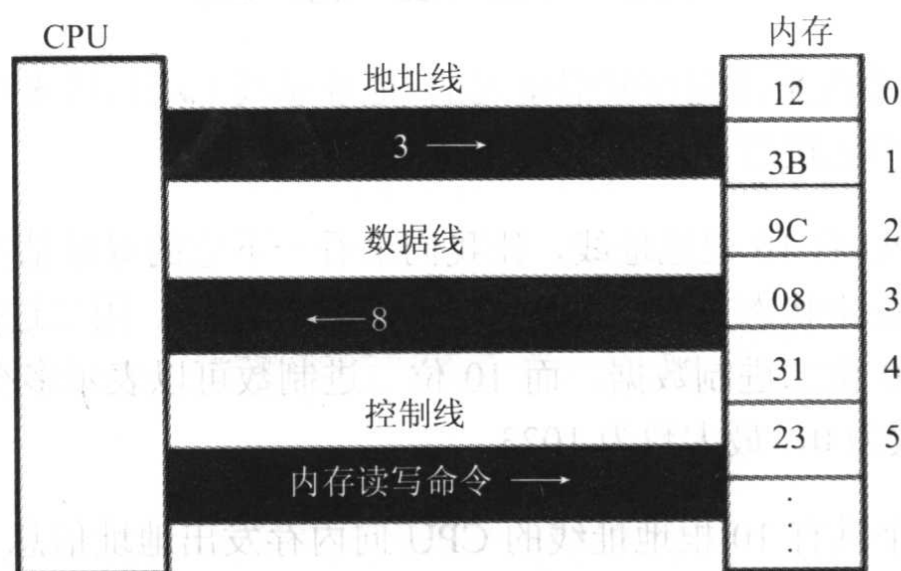
图 1.3 CPU 从内存中读取数据的过程
