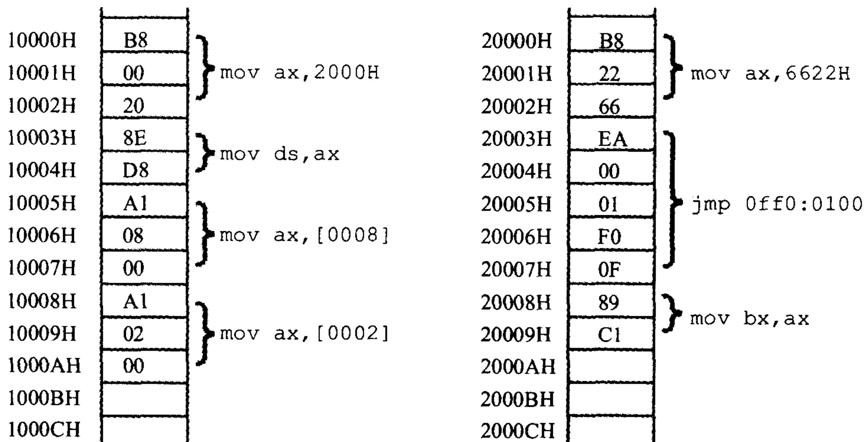
图 3.6 内存情况示意
