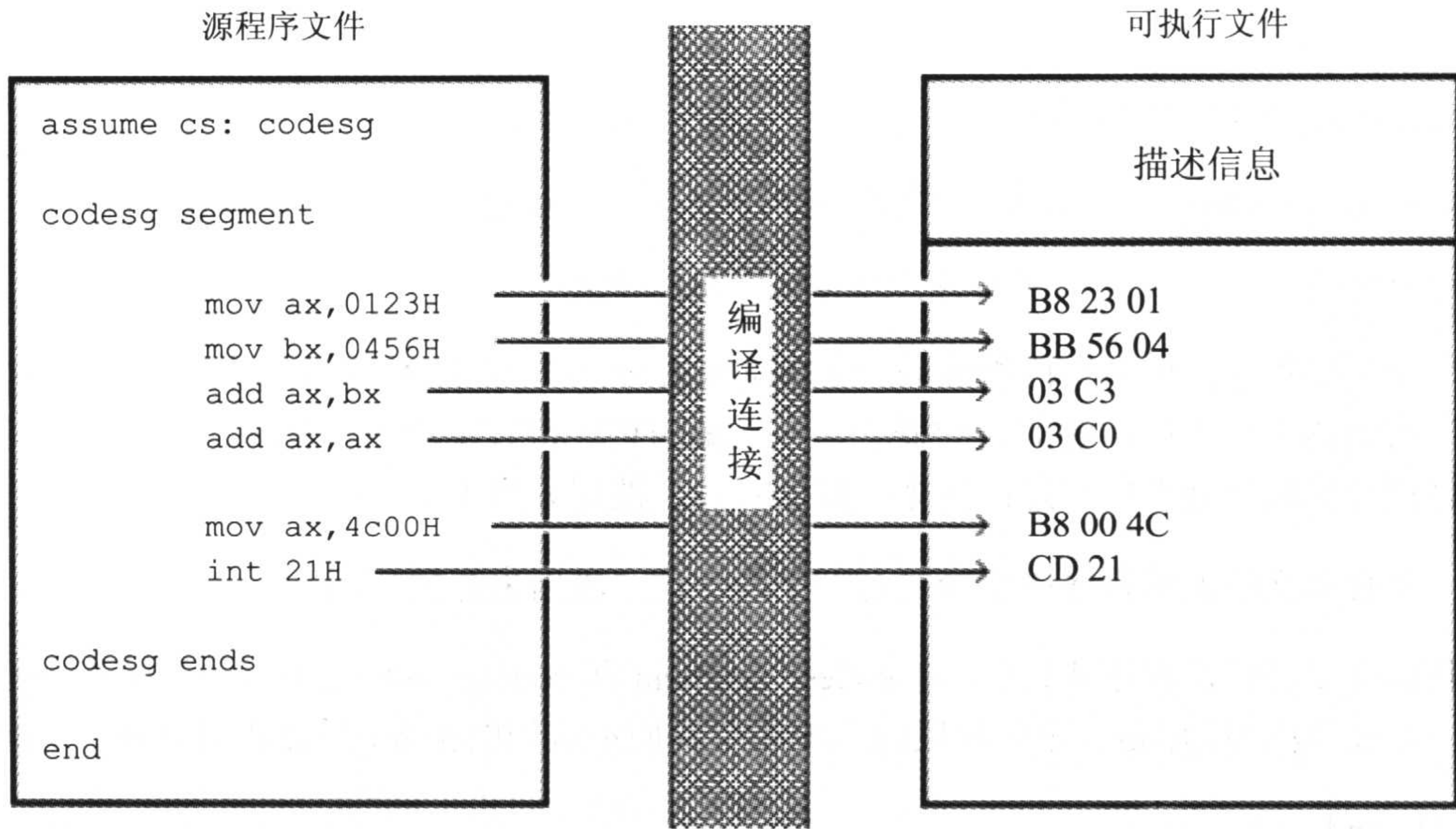
图 4.2 程序经编译连接后变为机器码
