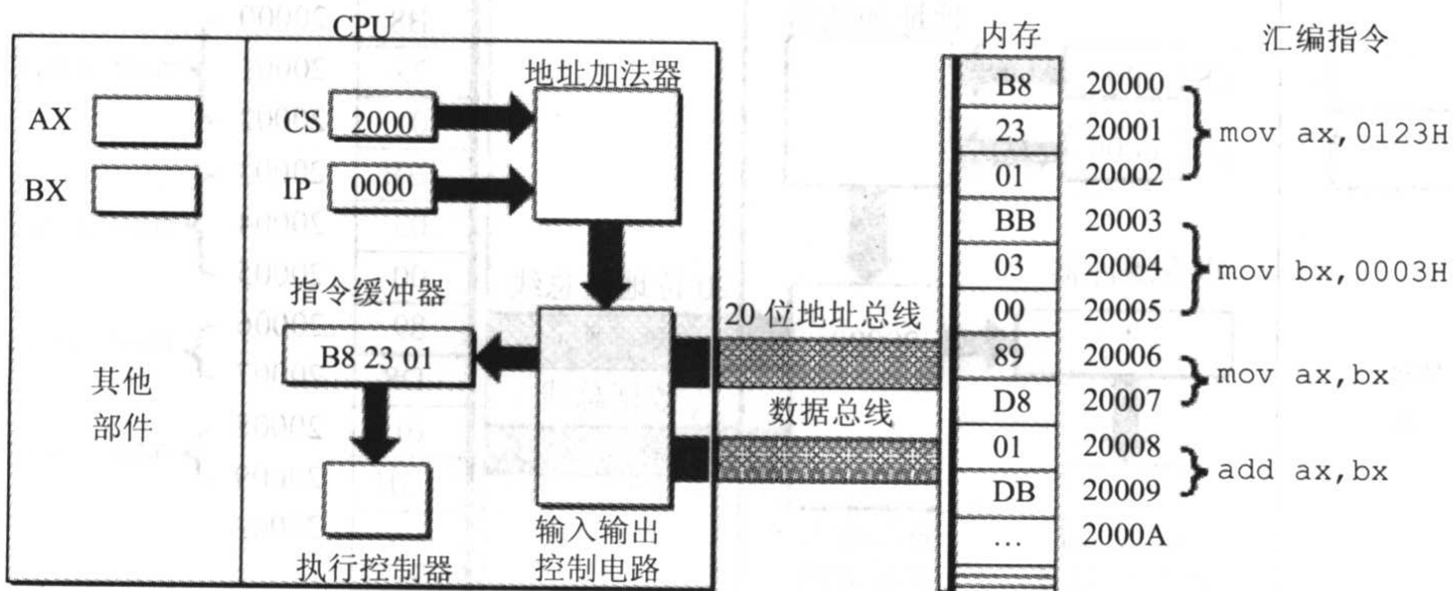
图 2.16 机器指令被送入指令缓冲器
