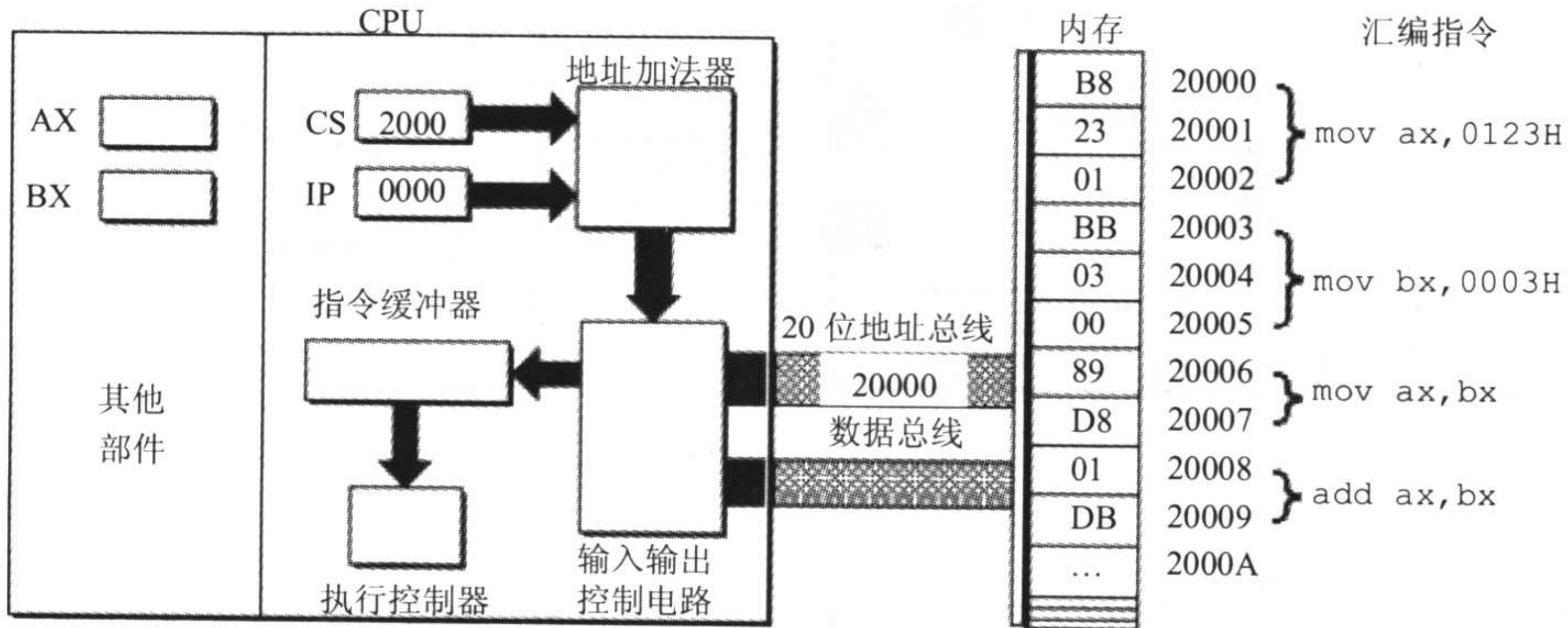
图 2.14 物理地址被送上地址总线
